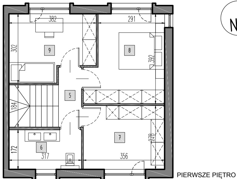
PIERWSZE PIĘTRO
