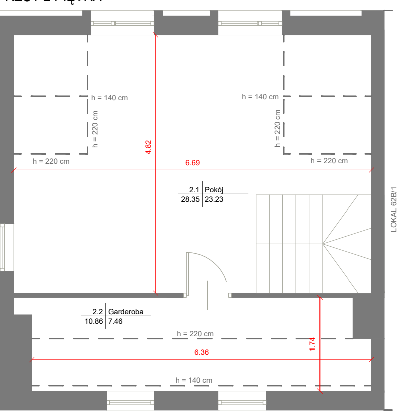
RZUT 2 PIĘTRA
