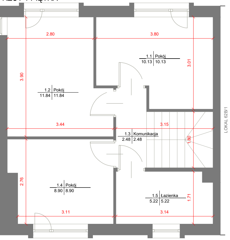
RZUT 1 PIĘTRA
